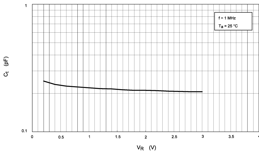
Fig. 9.3 C_t - V_R
