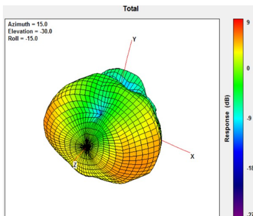
2690MHz
