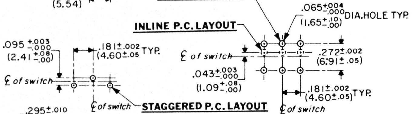
D.P. P.C. LAYOUT
