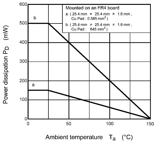
Fig. 7.11 P_D - T_a
