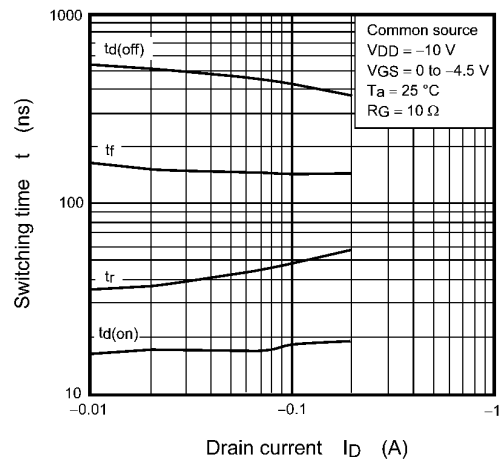
Fig. 7.10 t - I_D
