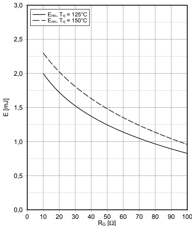
Schaltverluste Diode, Brems-Chopper (typisch) switching losses Diode, Brake-Chopper (typical) E_{rec} = f(R_G) I_F = 35 A, V_{CE} = 600 V
